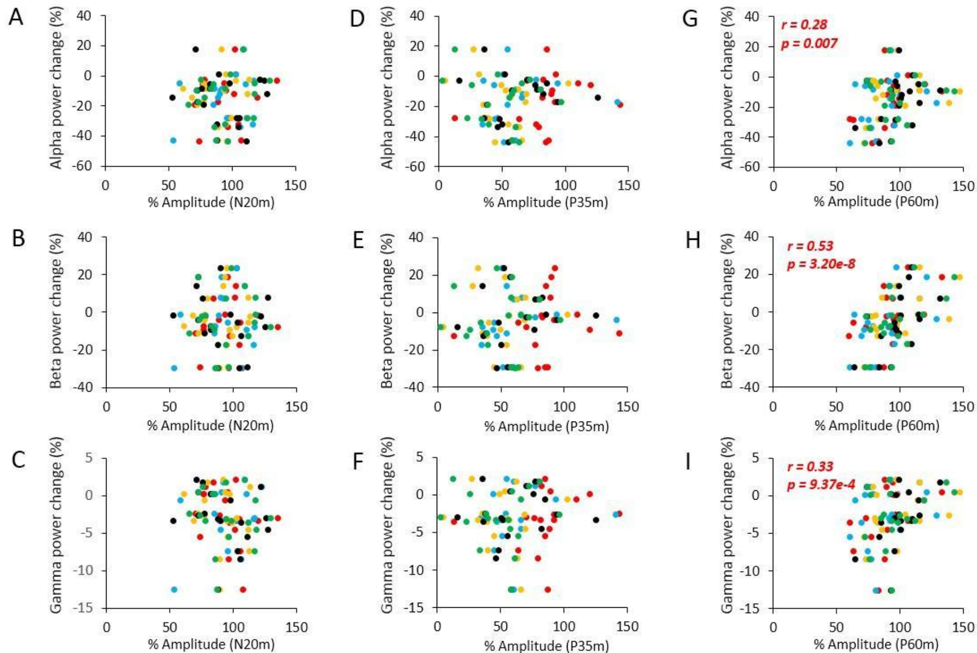
図3 PPD (N20m, P35m, P60m) と ERD ( \alpha , \beta , \gamma ) との関係
