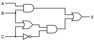
図 1 論理回路
