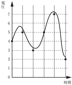
図 1 音の波形
